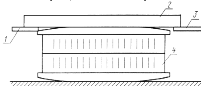
1 — щуп первый; 2 — поверочная линейка; 3 — щуп второй; 4 — блок
