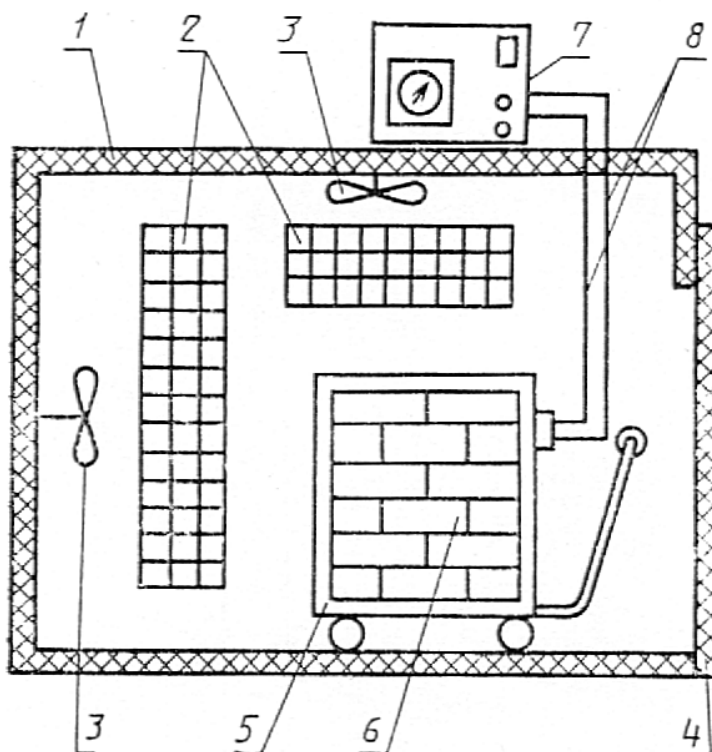
Схема испытания при использовании АДОЗО
