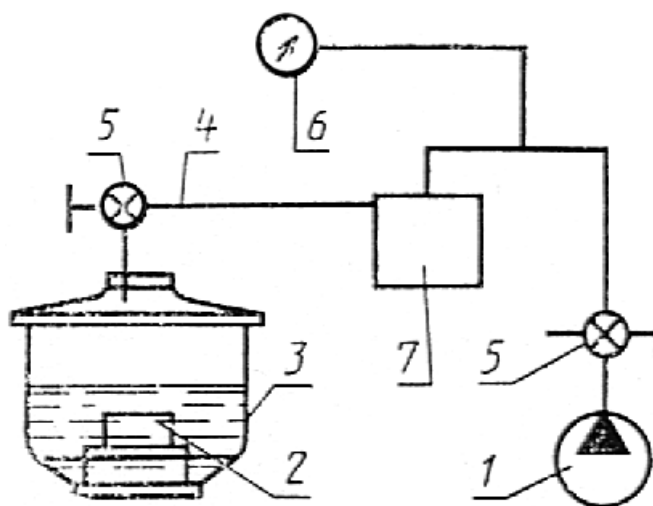
Схема установки для определения водопоглощения под вакуумом
