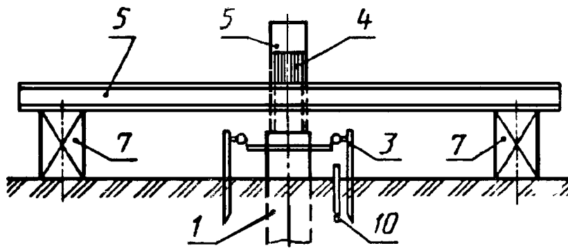
Схема установки для испытания грунтов статической горизонтальной нагрузкой
