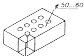
Рисунок А10 — Кирпич с 8 несвободными отверстиями (пустотность 11 %)
