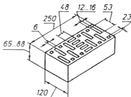
Рисунок А3 — Кирпич с 21 пустотами (пустотность 34 %, 45 %)
