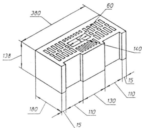
Рисунок А23 — Камень с пустотностью 45 %
