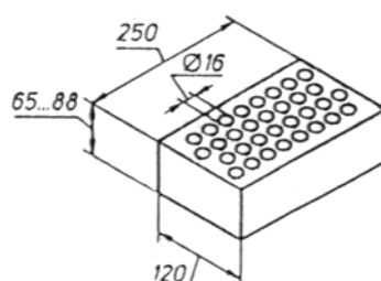
Рисунок А2 — Кирпич с 32 пустотами (пустотность 22 %)
