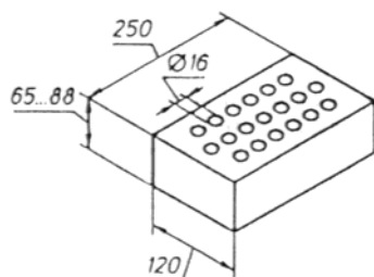
Рисунок А1 — Кирпич с 19 пустотами (пустотность 13 %)
