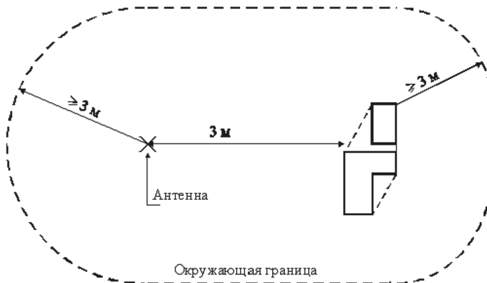
Рисунок 1 - Измерительная площадка
