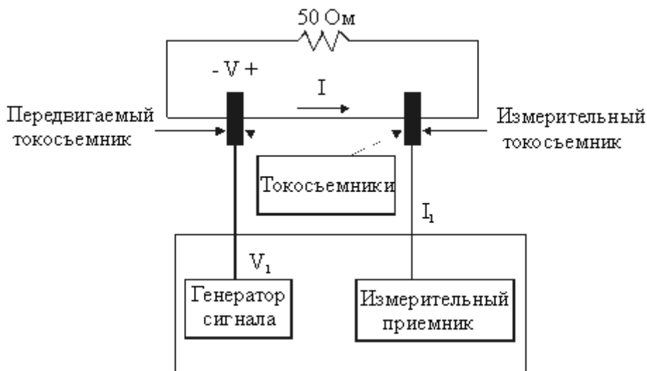
Рисунок Б.5 - Схема калибровки
