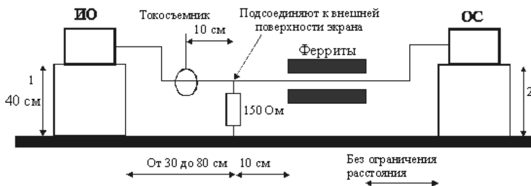
Рисунок Б.2 - Испытательная установка в соответствии с Б.1.2
