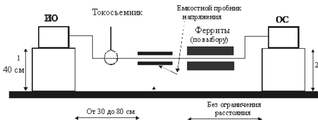
Рисунок Б.3 - Испытательная установка в соответствии с Б.1.3
