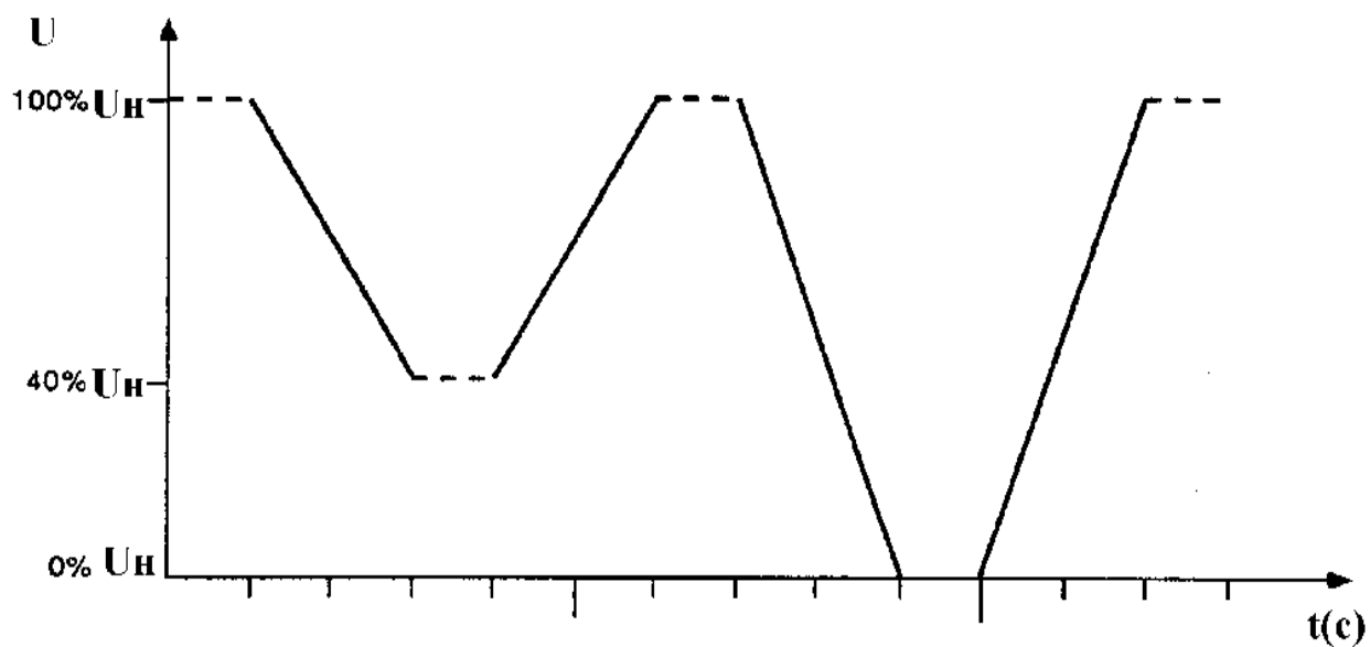
Рисунок 1 - Динамические изменения напряжения (провалы)
